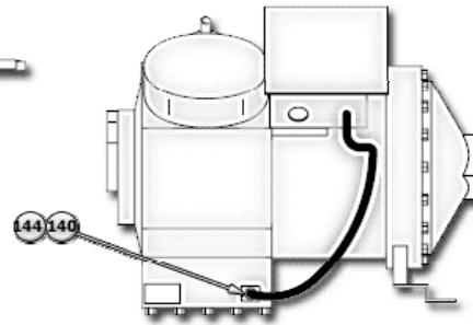
Semi-Hermetic 15-30 Ton
